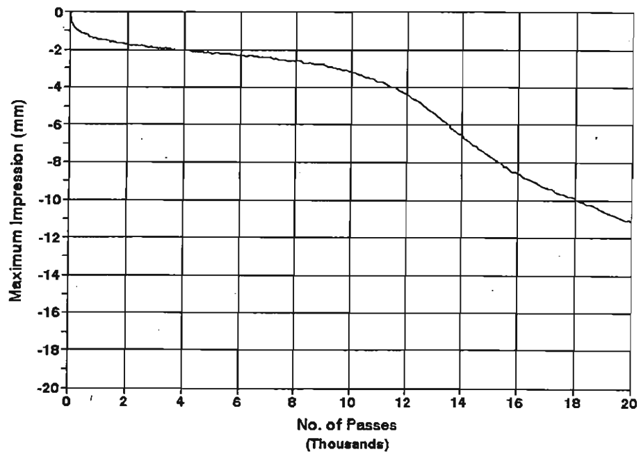
SITE2 L2 Temp. 45 C
