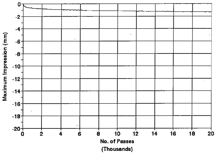
SITE6 L8 Temp. 50 C
