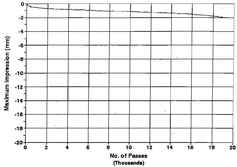
SITE2 L0 Temp. 45 C
