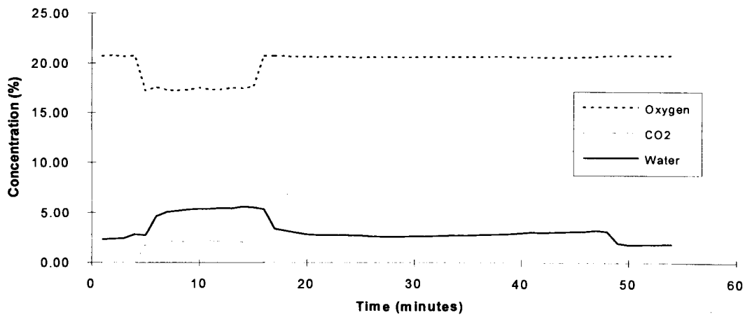
HFC -125 - Test 3
