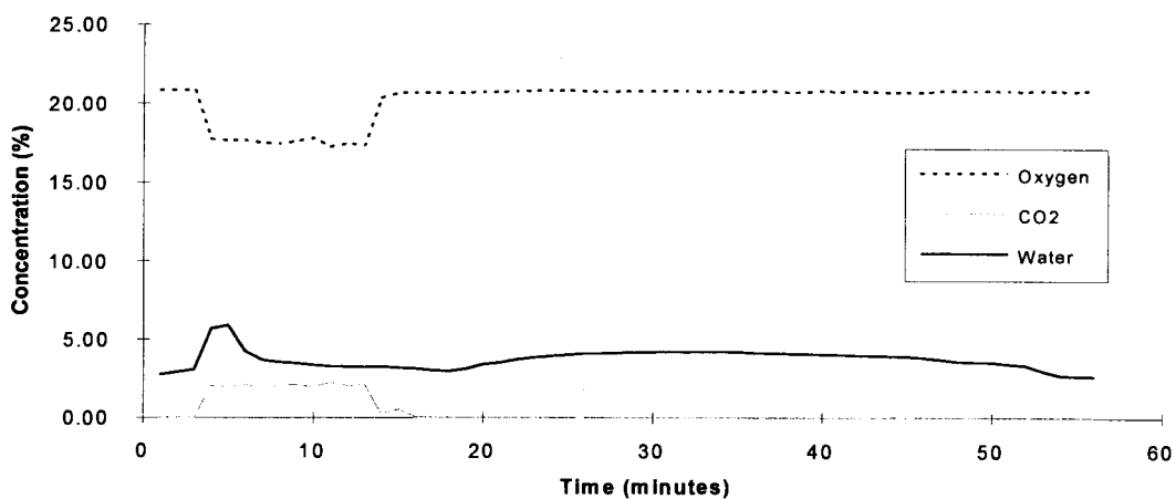
HFC -125 - Test 2
