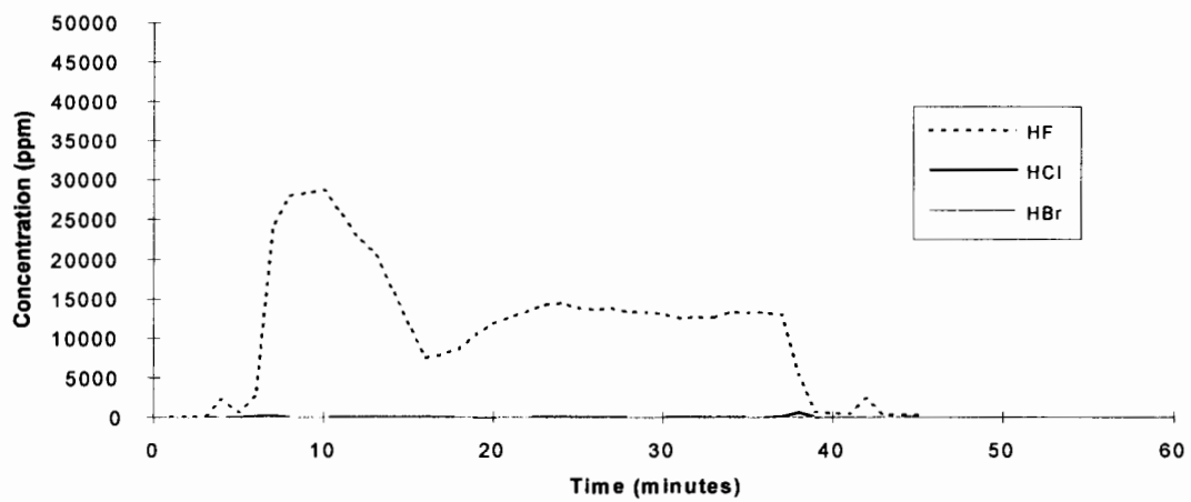
Perfluorohexane - Test 2
