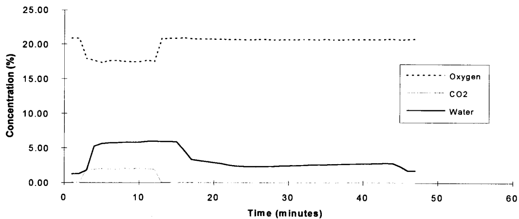
HFC -125 - Test 1
