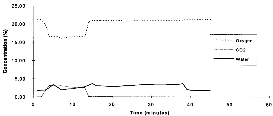
Perfluorohexane - Test 2
