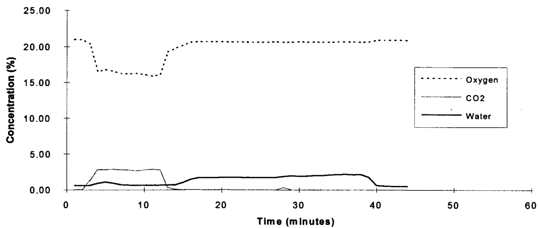
Perfluorohexane - Test 1
