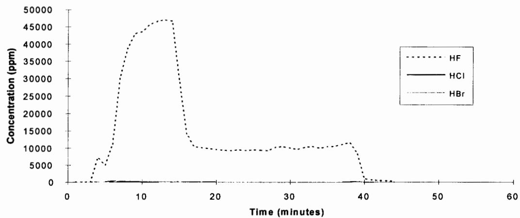
Perfluorohexane - Test 1
