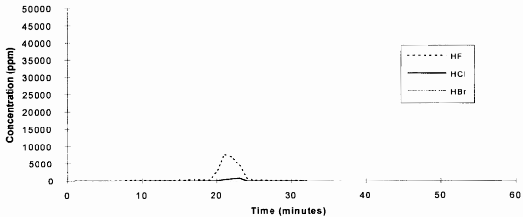
Halon 1301- Test 3
