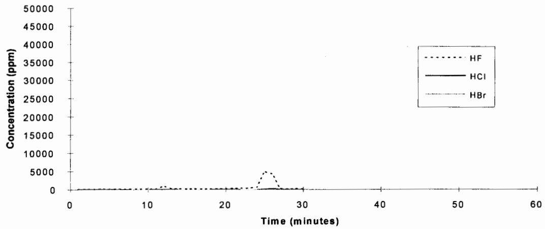
Halon 1301- Test 1
