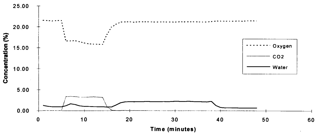
Perfluorohexane - Test 3
