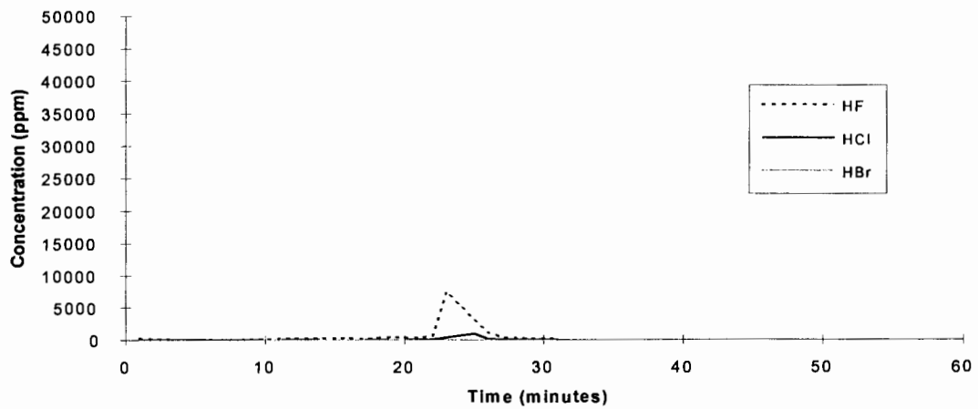
Halon 1301- Test 2
