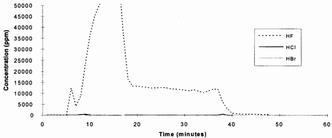
Perfluorohexane - Test 3
