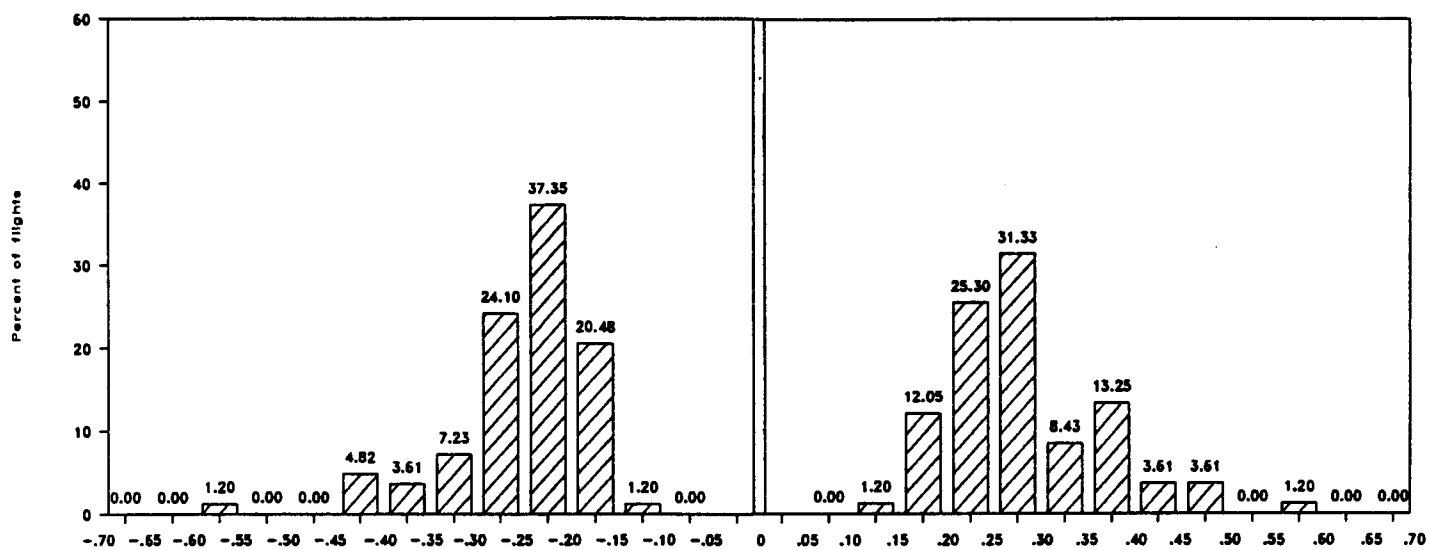
(b) a_n
