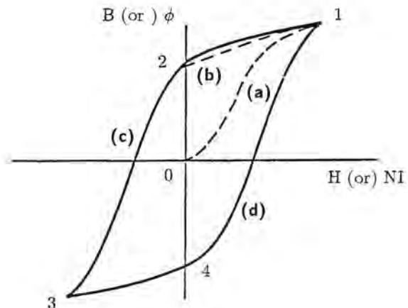
Fig. 18.19 B-H loop.
