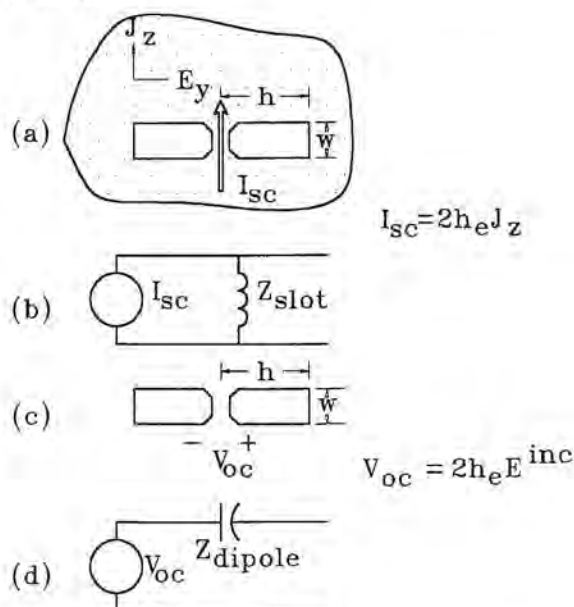
Fig. 12.18 Slot antenna.
