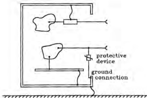
Fig. 18.36 Protected circuit.
