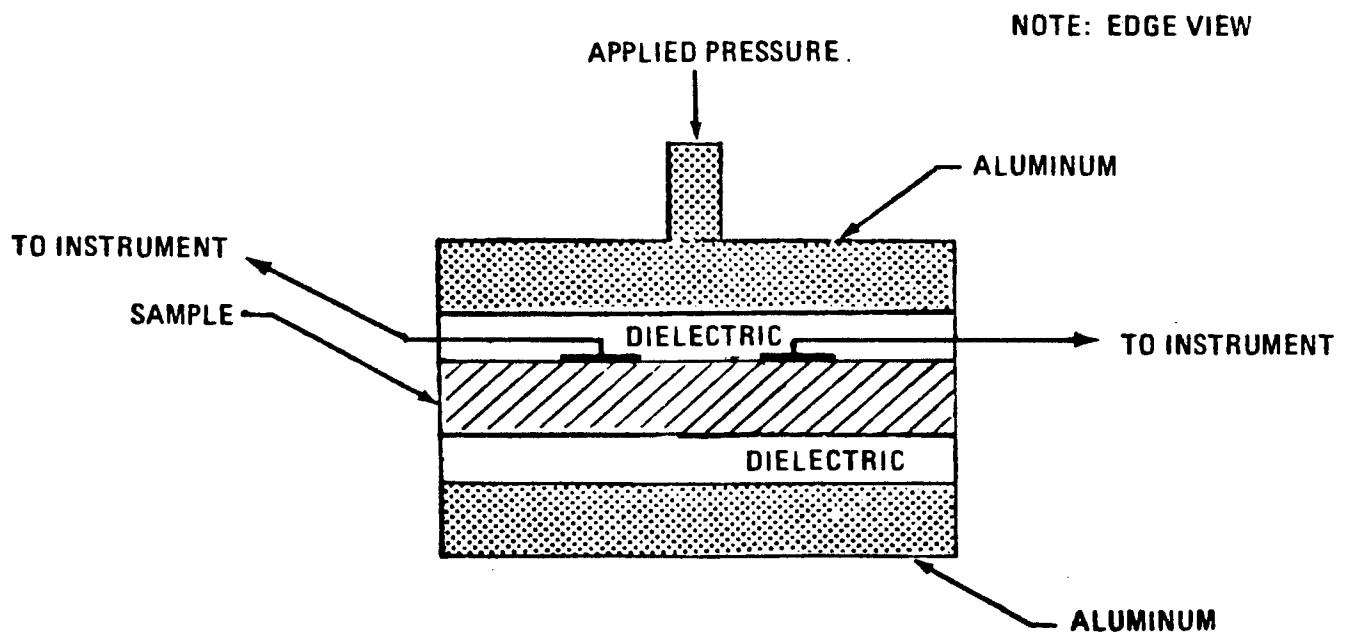
b. EDGE VIEW OF PROBE
