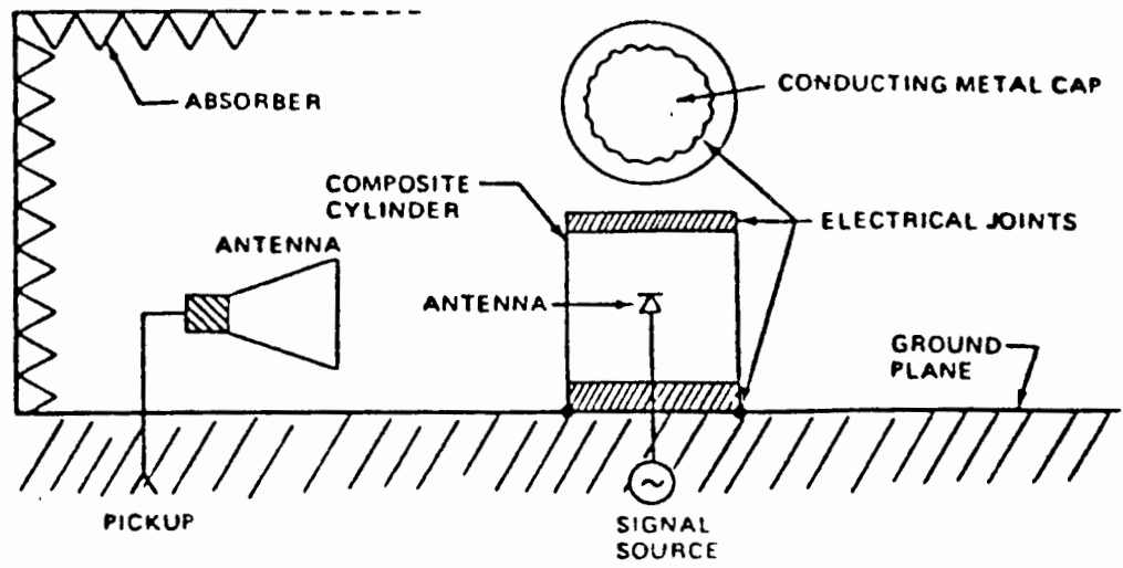
a. TEST SETUP
