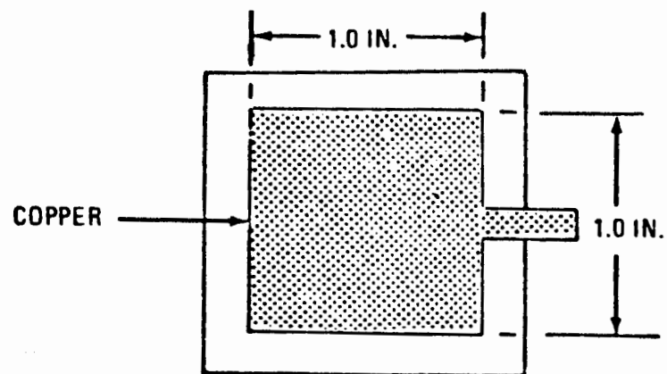
a. VOLUME PROBE
