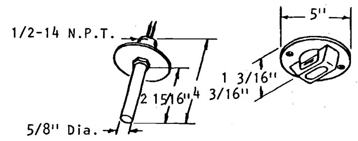
Detail A: Heat Detector
