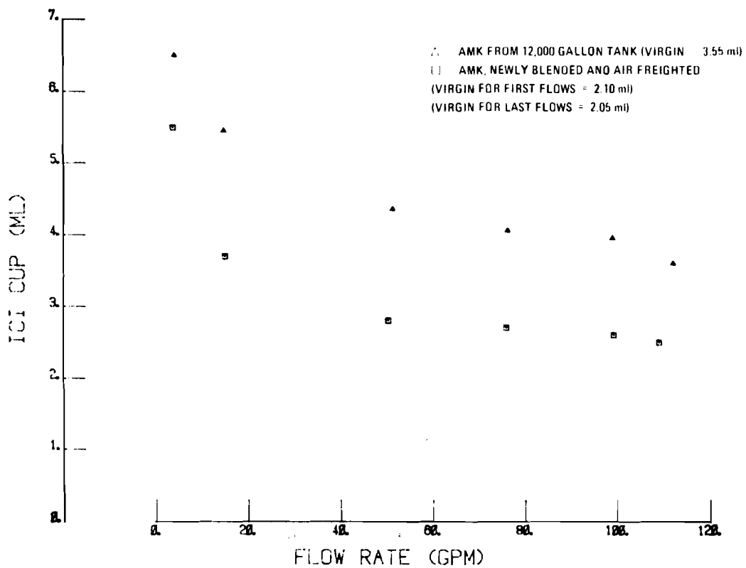
FIGURE 25. ICI CUP TEST, CONFIGURATION 1
