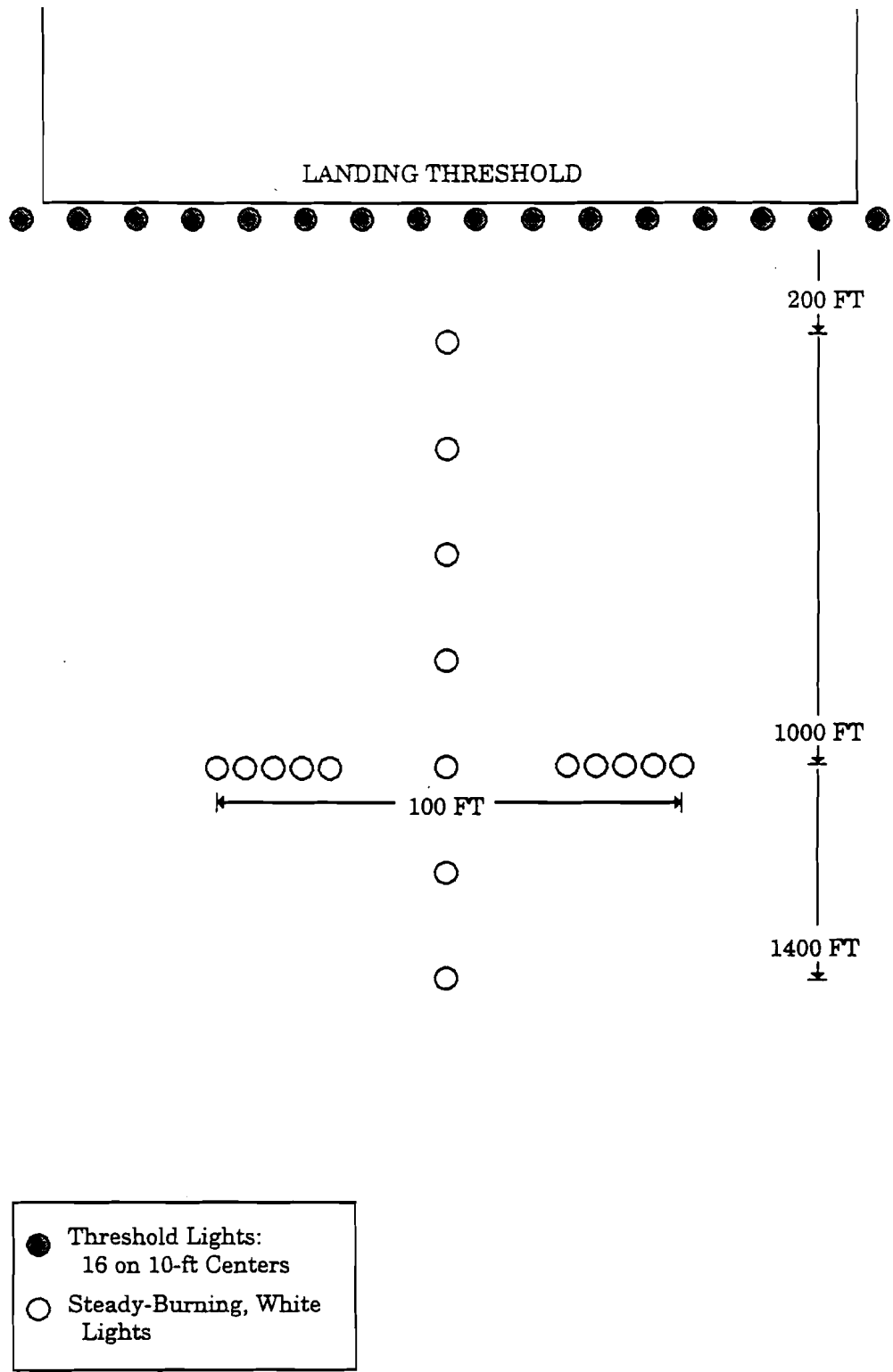
FIGURE 1. ICAO SIMPLE SINGLE SOURCE CENTERLINE ALS (CONFIGURATION C)
