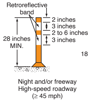
TUBULAR MARKERS
