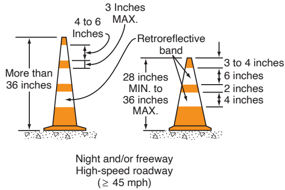
CONES
