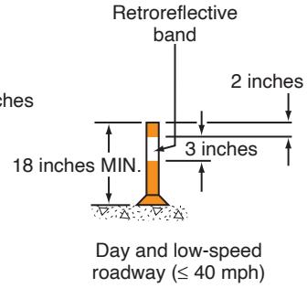
TUBULAR MARKERS
