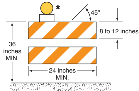
TYPE 2 BARRICADE **
