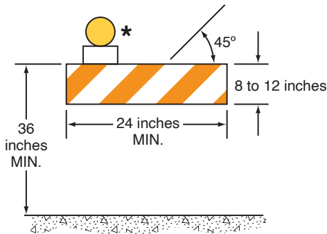
TYPE 1 BARRICADE **
