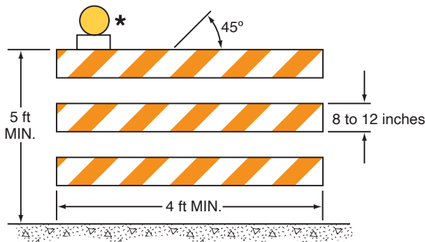
TYPE 3 BARRICADE **
