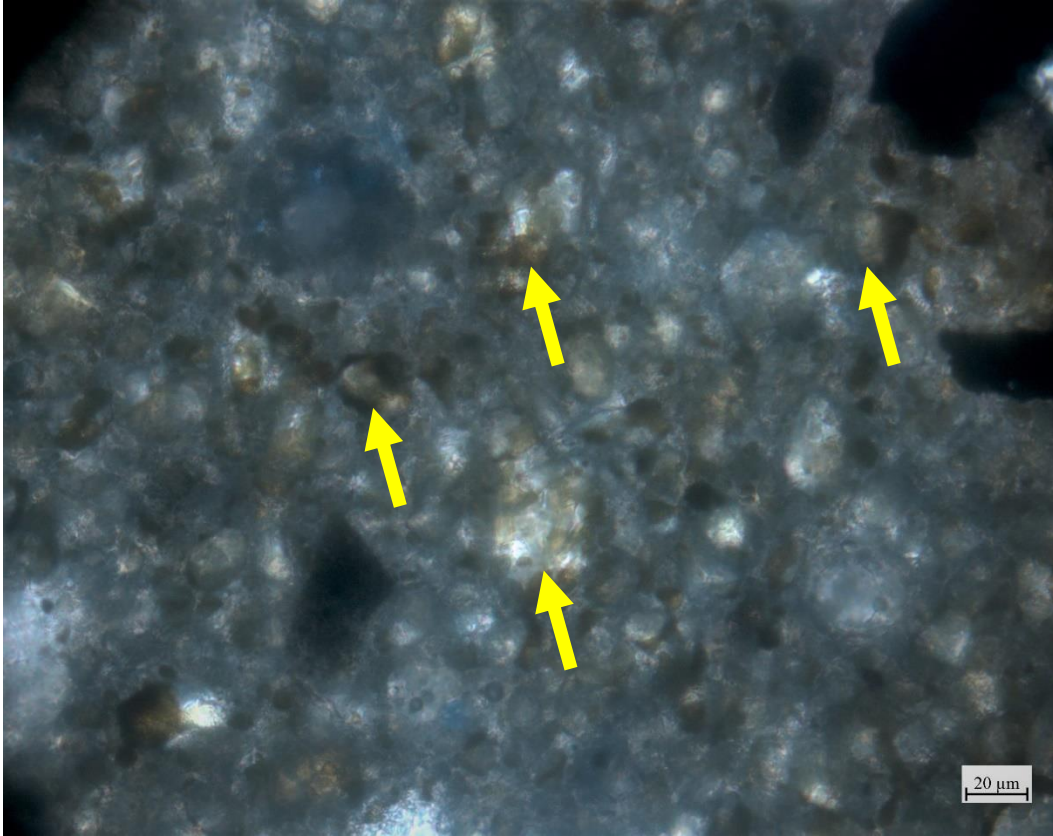
(Yellow arrow: unhydrated cement particles)
