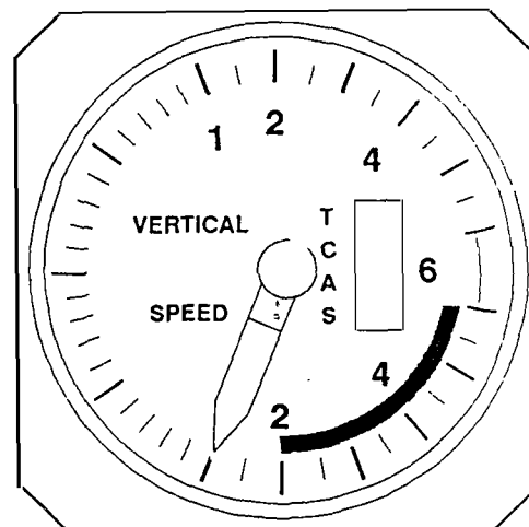
(d) Preventive MONITOR VERTICAL SPEED.
