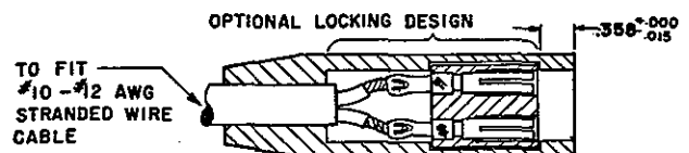
RECEPTACLE, g&amp;h Assembled, Style 12
