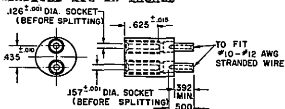
g - INSERT ASS'Y
