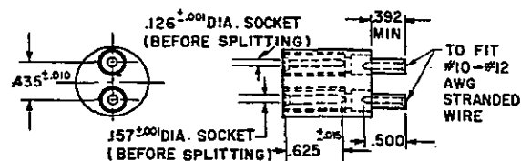
c - INSERT ASS'Y
