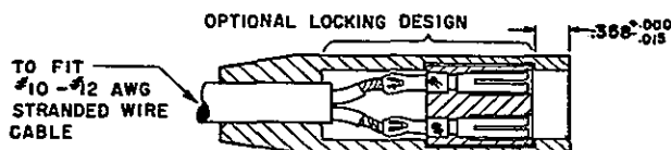
RECEPTACLE, g&amp;h Assembled, Style 12
