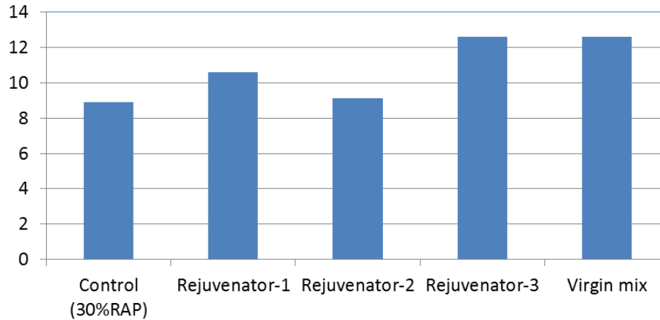
Hamburg Rut depth (mm)
