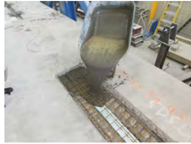
b. Pouring LMC
