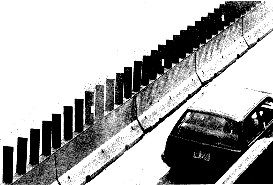
Glare blades
