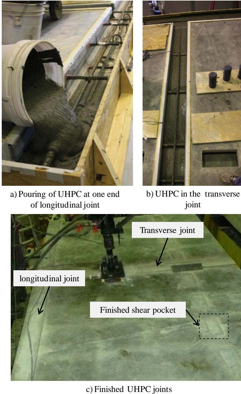
Figure 9 UHPC joint pour
