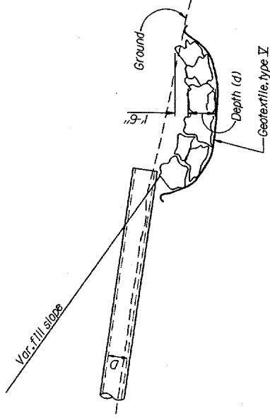
ELEVATION
