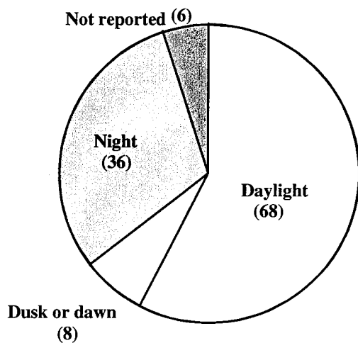
IMC
