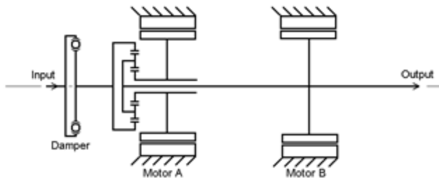
1-Mode EVT Arrangement (Input-Split EVT)
