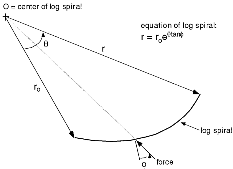
(b) Log spiral.
