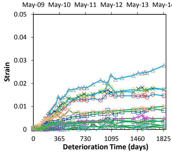
(d) Horizontal DEMEC Strains in Joint
