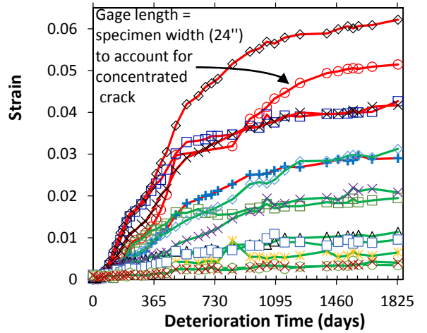
(d) DEMEC Strains in Joint
