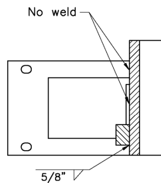
D-D
