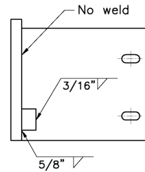
D-D
