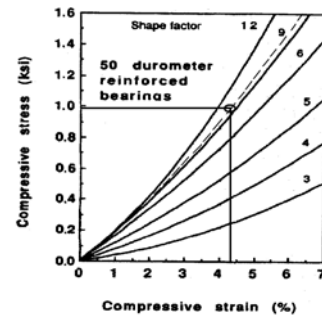
(LRFD 14.7.5.3.3-1)
