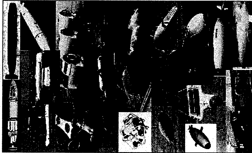
UUVs (> 70 Vehicles)
