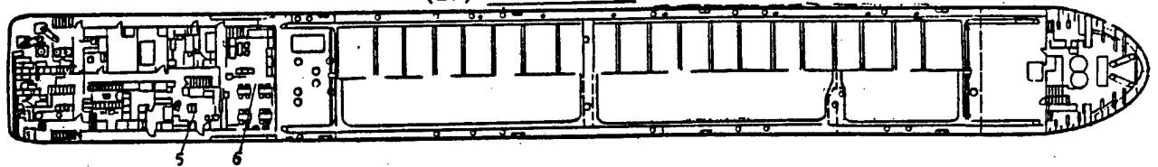
(20) Полубак
