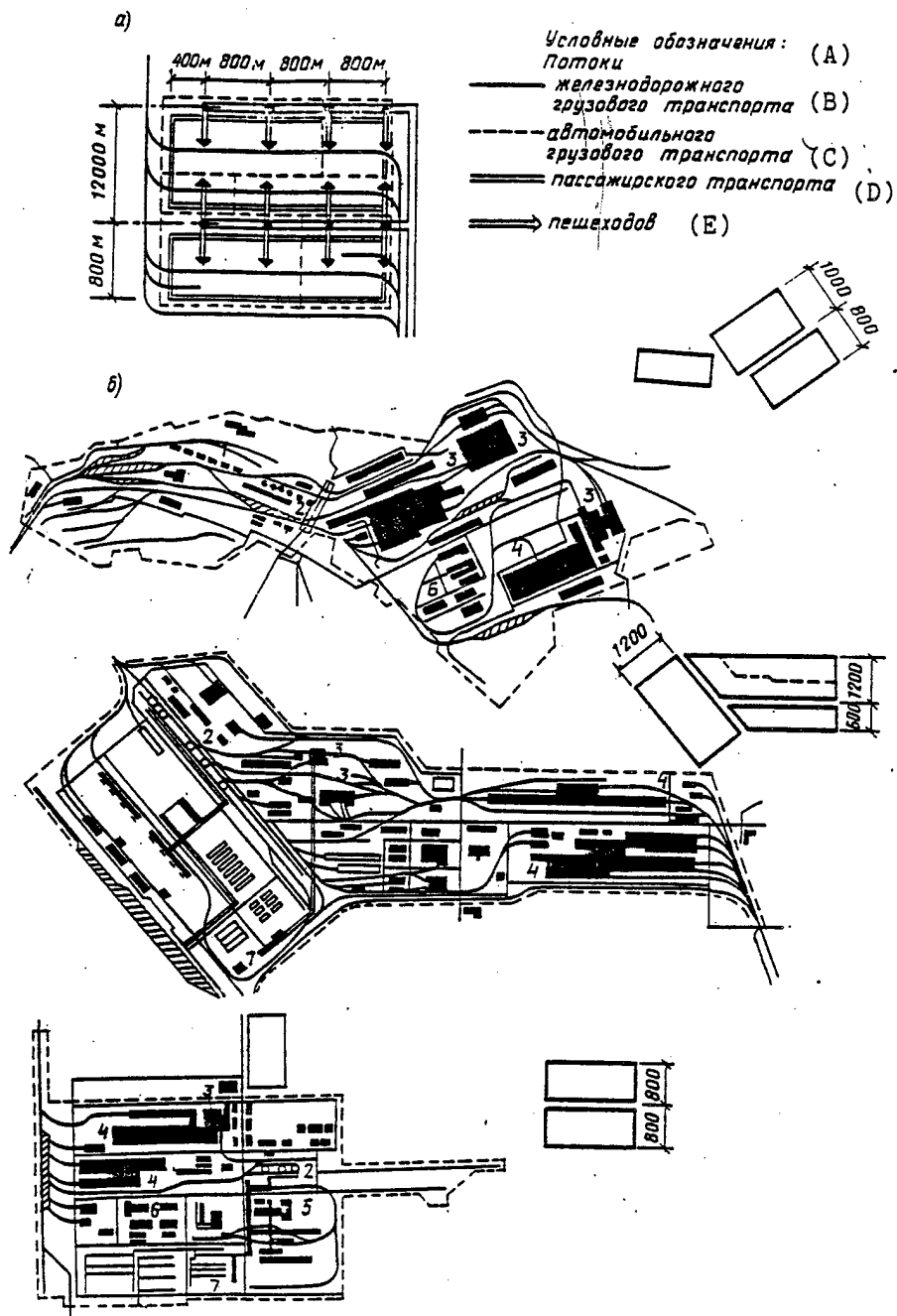
Рис. 1. Деление на панели территории действующих предприятий по условиям обслуживания пассажирским транспортом а — принципиальная схема организации планировочной структуры предприятия; б — пример; 1 — коксохимическое производство; 2 — доменное производство; 3 — сталеплавильные цехи; 4 — прокатные цехи; 5 — аглофабрика; 6 — ремонтно-механические цехи; 7 — складское хозяйство
