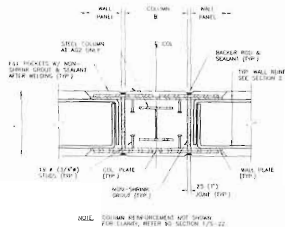
AG1 & AG2 SECTION
