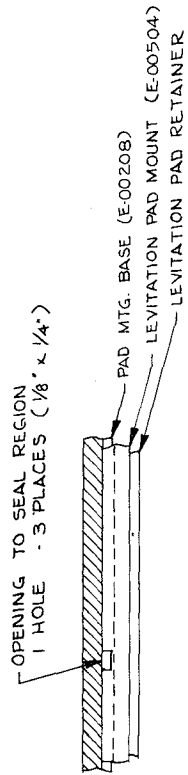
DETAIL C SCALE: 1/1
